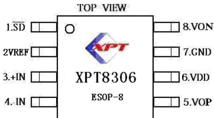
图为 XPT8306 ESOP8 封装的管脚分布图。
